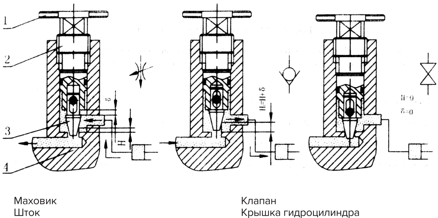
Рис. 18.5. Устройство и принцип работы клапана регулирования скорости работы.
